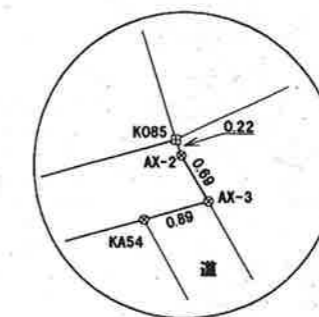
拡大図1/100
